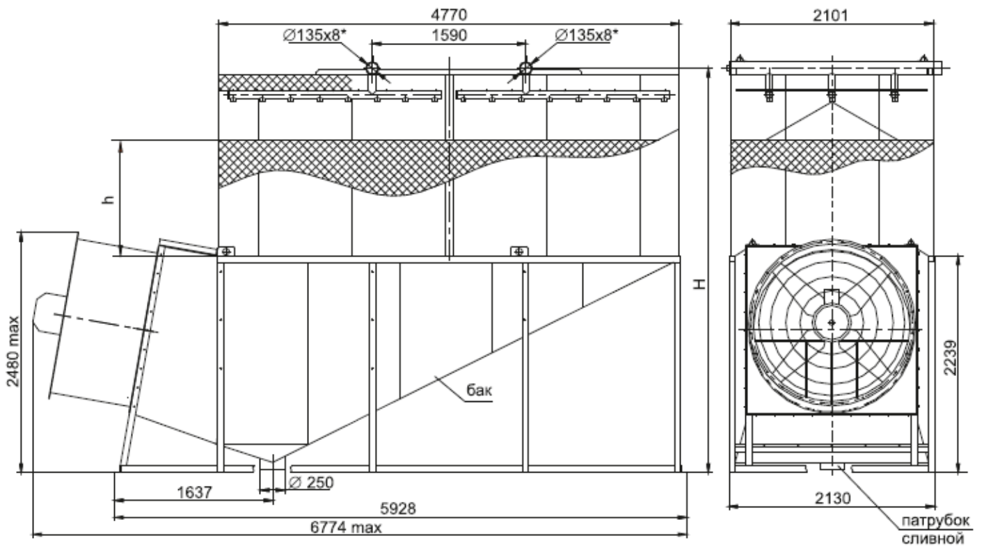
Рис. 9. Градирня ЕВРОМАШ-1650
