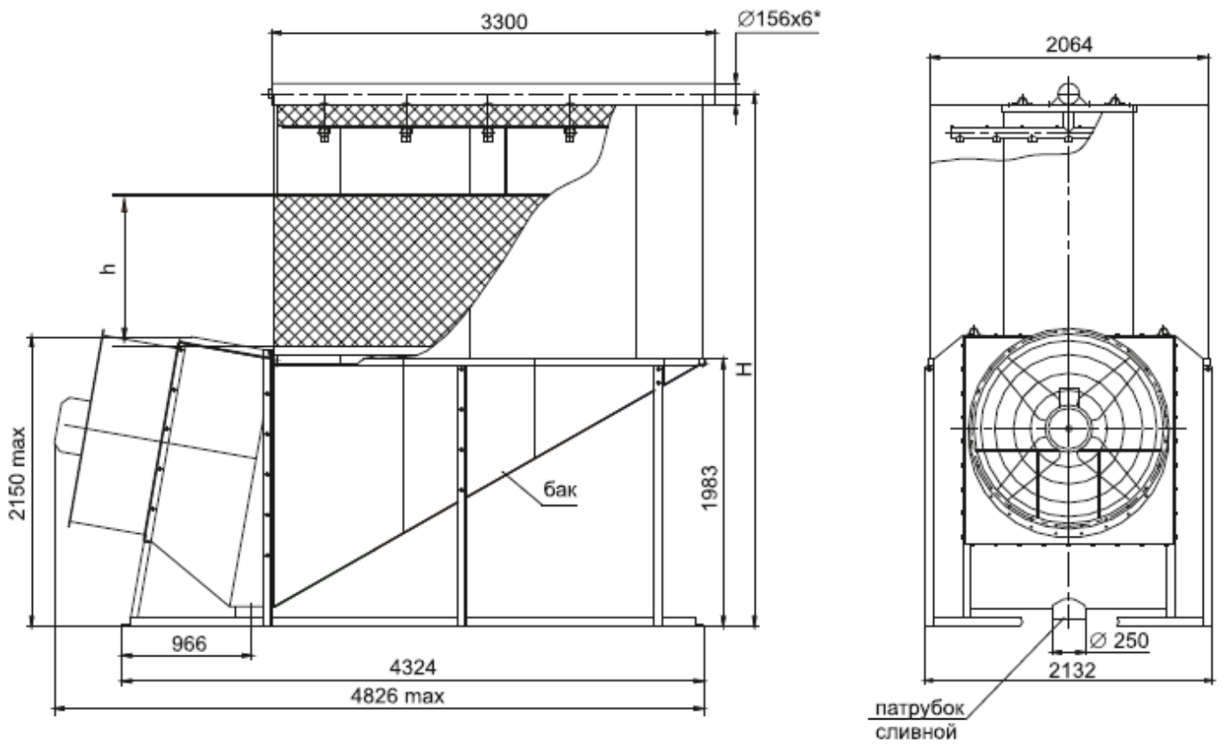
Рис. 8. Градирня ЕВРОМАШ-1000
